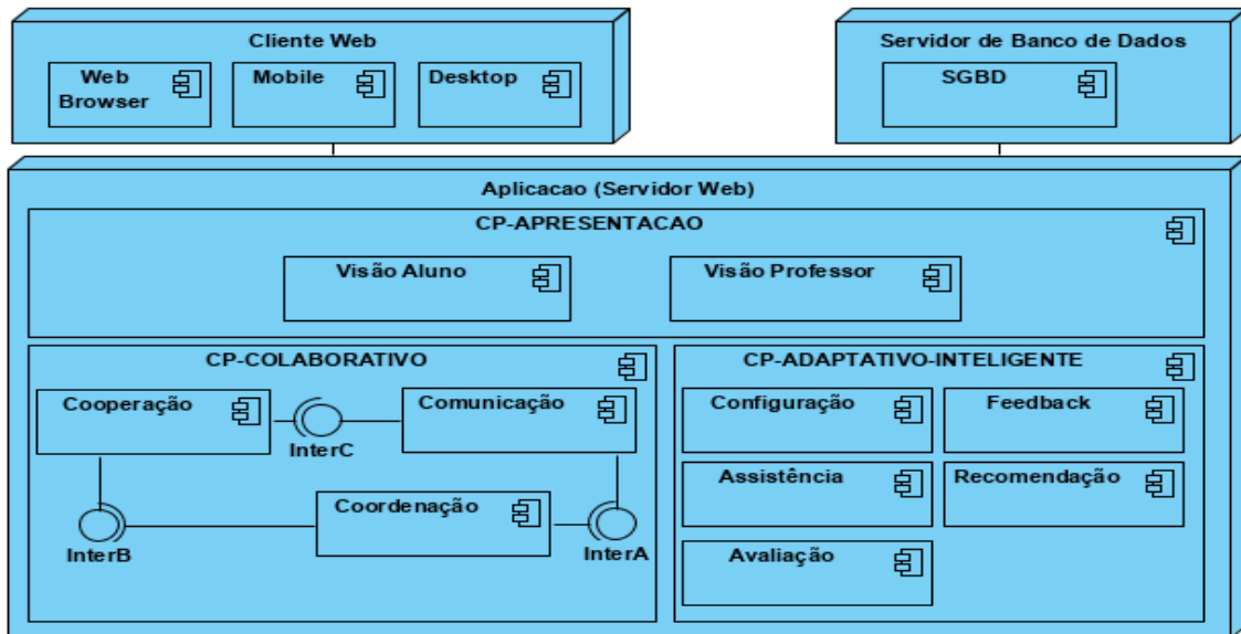
Figura 2 - Diagrama de arquitetura do ambiente computacional proposto.
