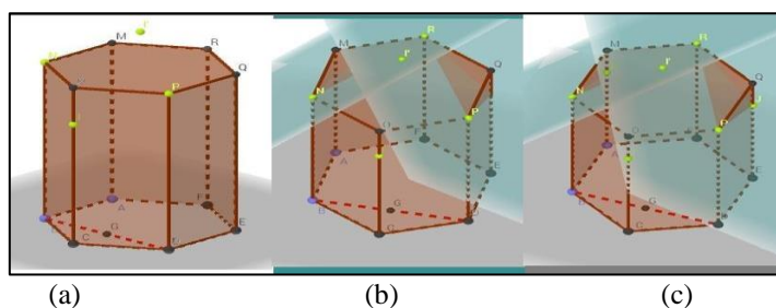
Figura 4. (a) Vértices de um losango. (b) Construção dos planos que contém os outros dois losangos. (c) Determinação dos últimos vértices do alvéolo.
